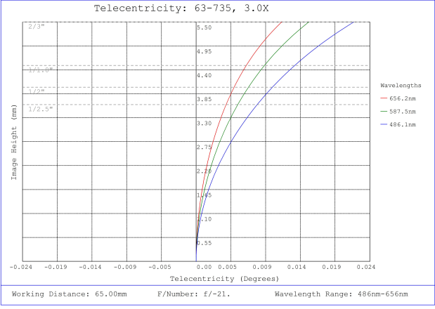
#63-735, 3X, 65mm WD CompactTL™ Telecentric Lens, Telecentricity Plot
